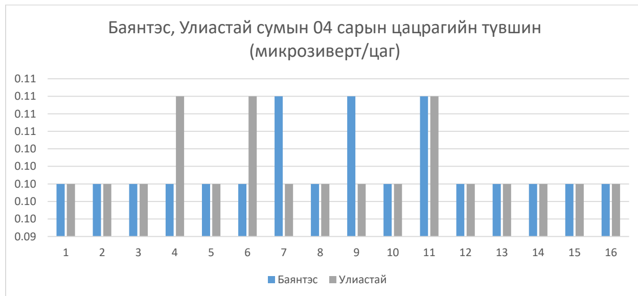
Зураг 1 . Цацрагийн өдрийн дундаж агууламж 04 сар
